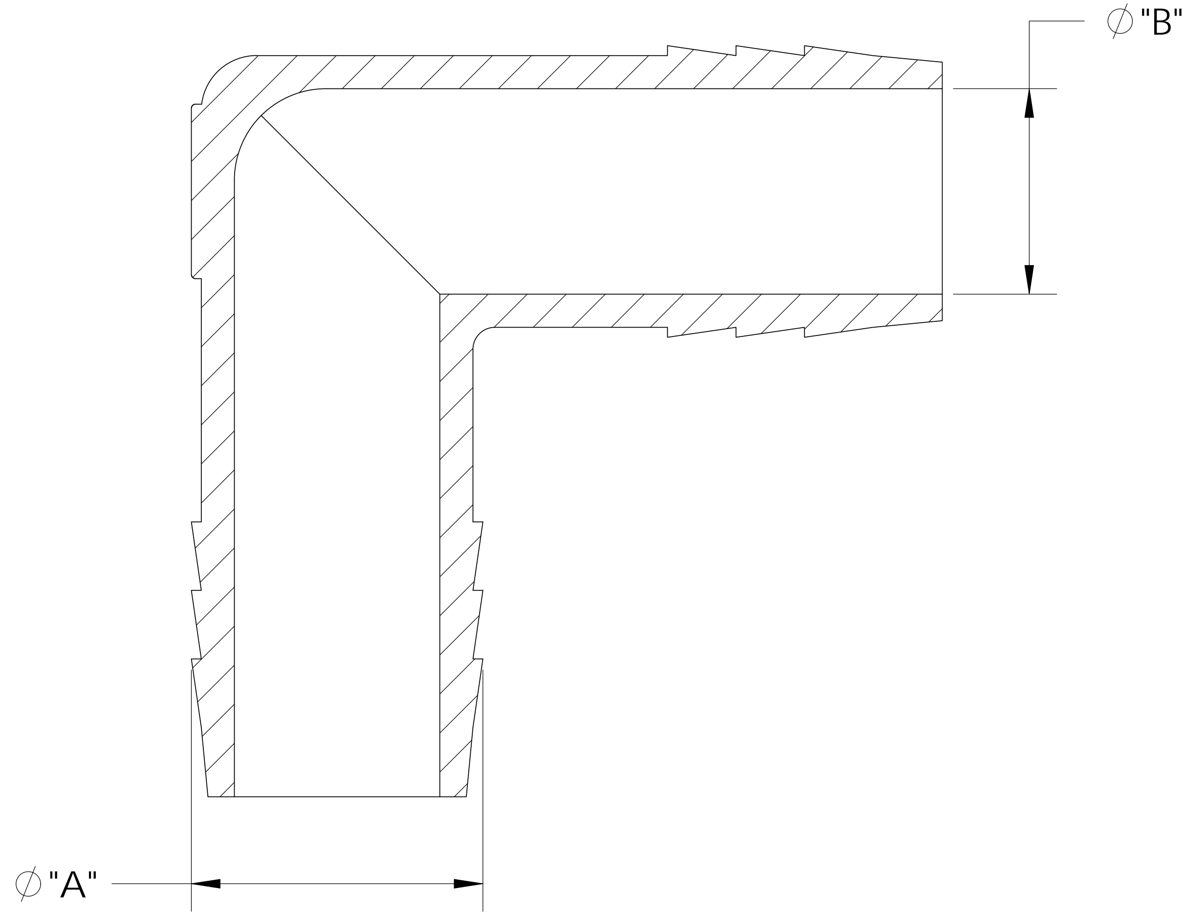
SECTION A-A
